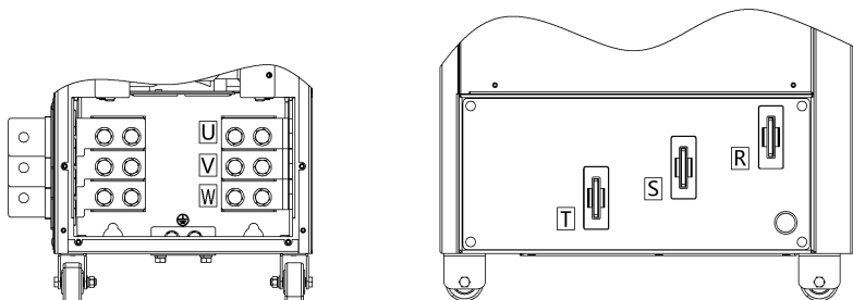
(j) 主回路功率端子 (3T0425-3T0950G)
