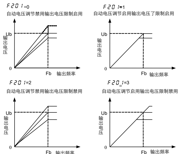
图 6.5 AVR 功能示意图
