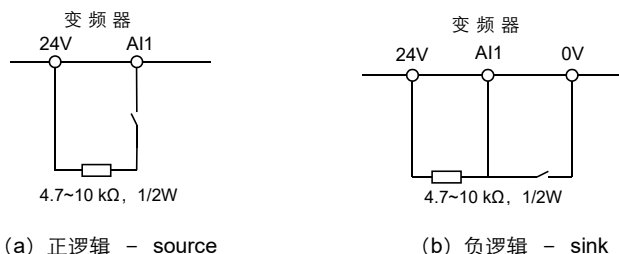
图 4.7 AI1 配置为逻辑输入端子时的接线图
