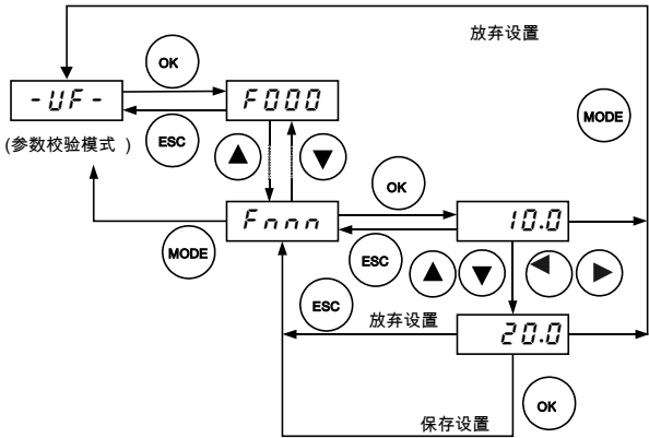
图 5.6 参数校验模式导航
