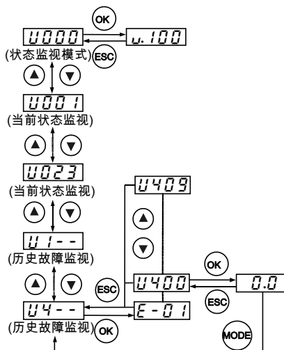
图 5.5 状态监视模式导航
