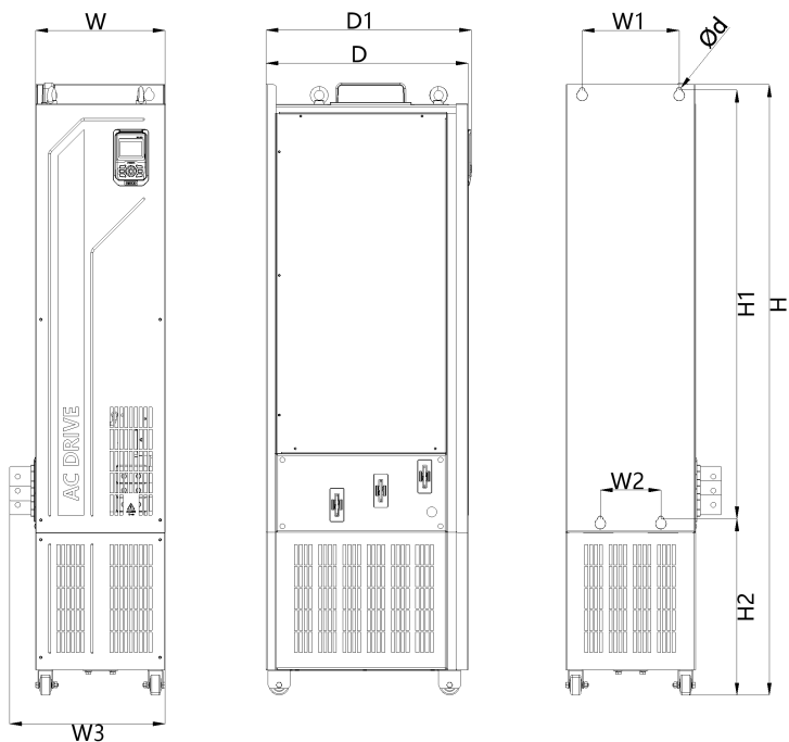
图 3.5 外形及安装尺寸示意图 (3T0425F -3T0950GF 含交流输出电抗器)
