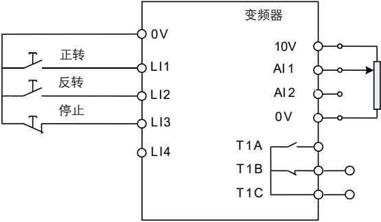
图 5.8 3 线控制（负逻辑）接线示意图
