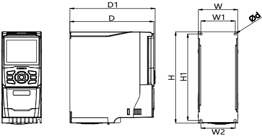
图 3.2 外形及安装尺寸图 (3T0032B 及以下)
