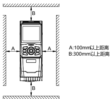
图 4.2 单台安装间距要求
