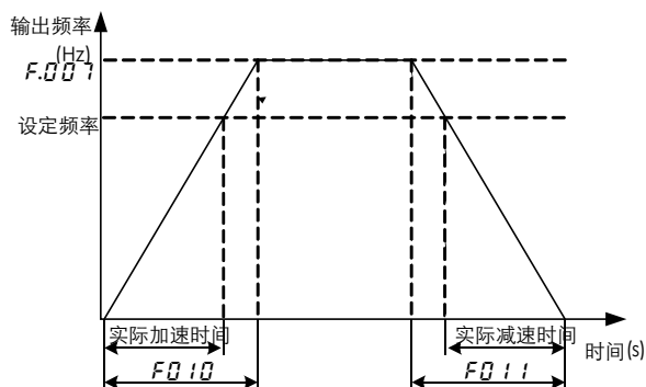
图 6.3 加速时间和减速时间定义
