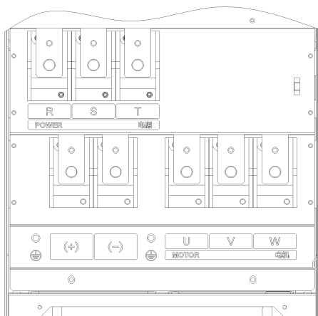
(i) 主回路功率端子 (3T0305-3T0380)
