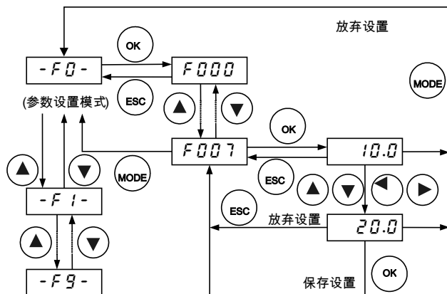
图 5.4 参数设置模式导航
