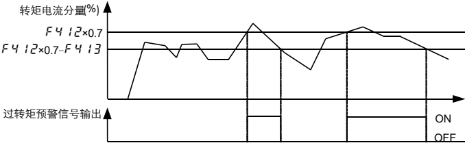
a) 过转矩/过电流报警输出示意图
