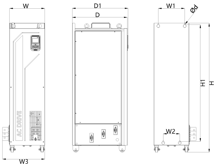
图 3.4 外形及安装尺寸示意图 (3T0425 -3T0950G 不含交流输出电抗器)
