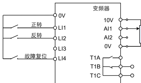
图 5.7 2 线控制接线示意图（负逻辑）
