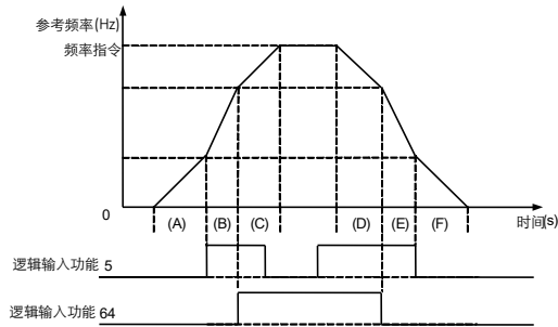
图 6.32 通过逻辑输入切换加速/减速曲线
