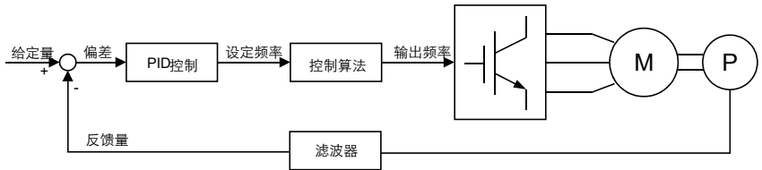
图 6.36 PID 控制基本原理框图
