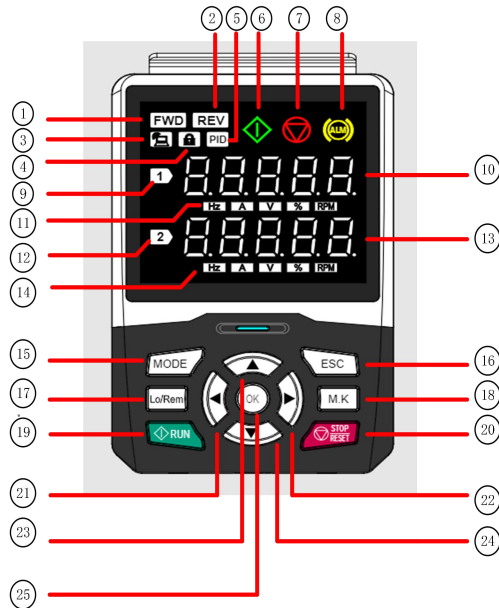
图 5.1 操作面板外形
