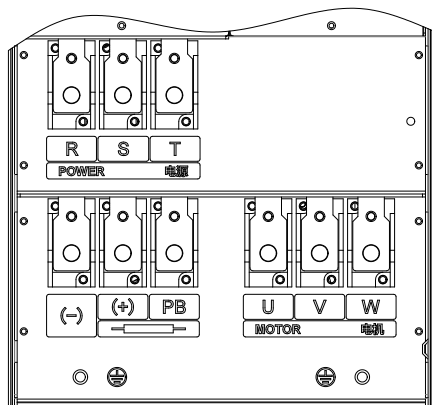
(h) 主回路功率端子 (3T0180-3T0260)
