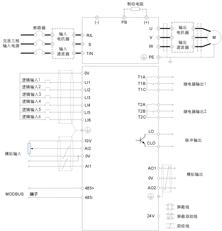
(a) 3T0032B 及以下标准接线图
