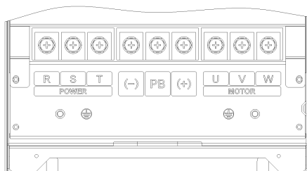
(f) 主回路功率端子 (3T0115)
