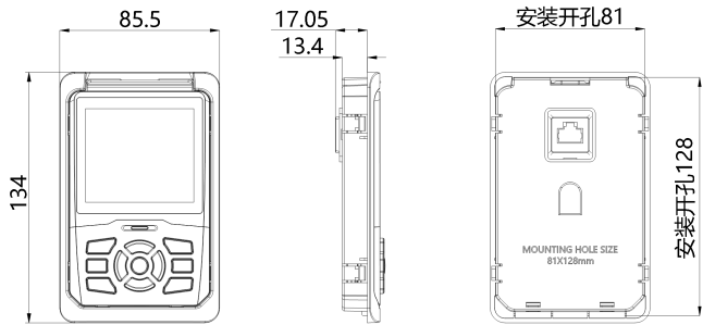
图 3.6 外引面板及托盘尺寸示意图
