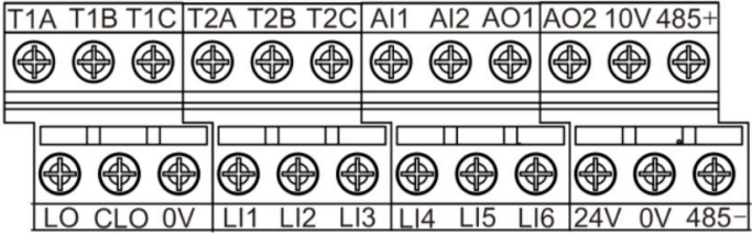
(a) 控制端子（3T0032B 及以下）
