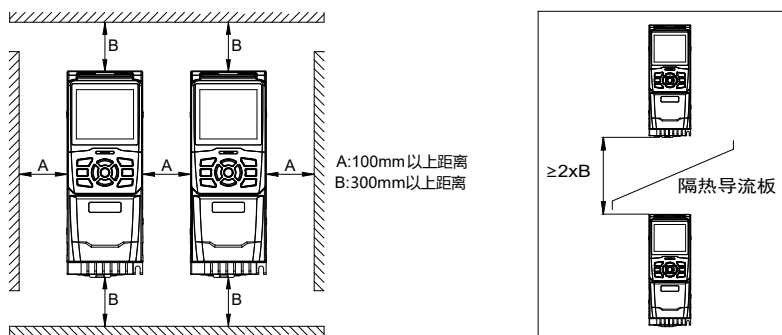
图 4.3 多台安装间距要求
