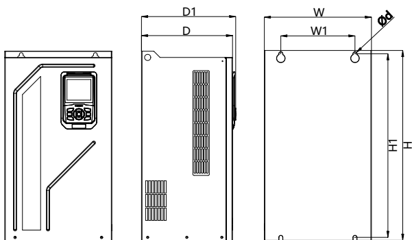
图 3.3 外形及安装尺寸示意图 (3T0038B -3T0380)
