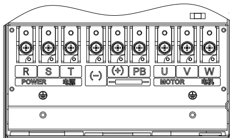
(g) 主回路功率端子 (3T0150)
