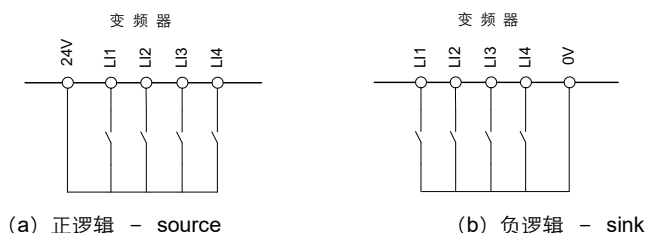
图 4.8 逻辑输入端子接线图
