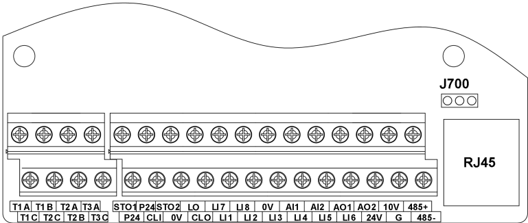
(b) 控制端子（3T0038B 及以上）
