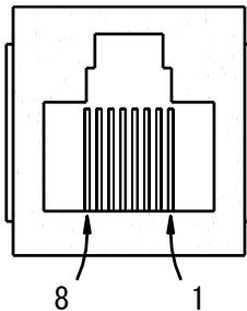
图 A.1 RJ45 正视图
