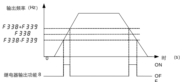
图 6.14 继电器输出-频率检出 2 示意图
