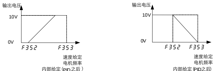
图 6.19 F352 和 F353 设置示意图
