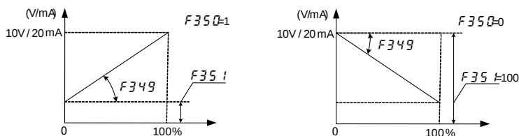
图 6.18 参数 F349 、 F350 和 F351 设置示意图
