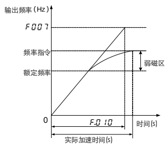
图 6.29 S 型曲线 2
