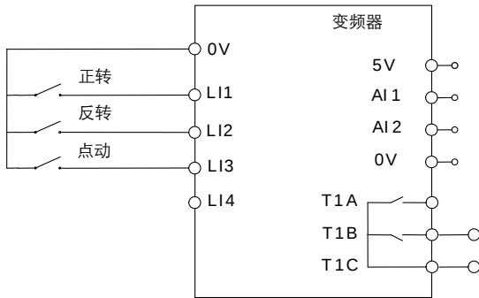
图 5.11 点动控制接线示意图
