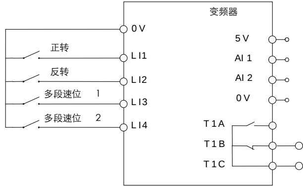
图 5.10 多段速控制接线示意图
