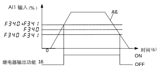
图 6.15 继电器输出-AI1 输入检出示意图
