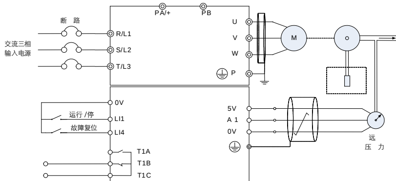
图 5.38 PID 外部连接示例
