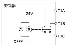
a)继电器 OFF 状态
