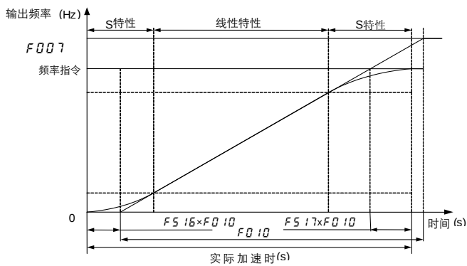
图 6.28 S 型曲线 1
