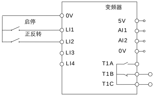
(6) 2 线控制模式 2-自锁开关（电平）正反转控制示例 6：（负逻辑）
