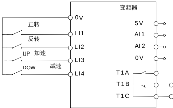
图 5.9 UP/DOWN 加减速接线示意图
