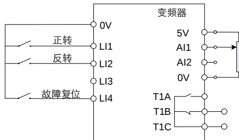
图 5.7 2 线控制接线示意图
