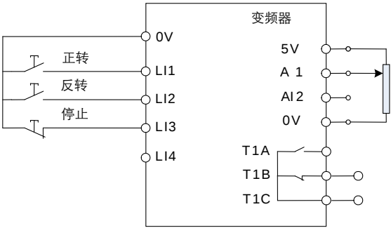
图 5.8 3 线控制（负逻辑）接线示意图
