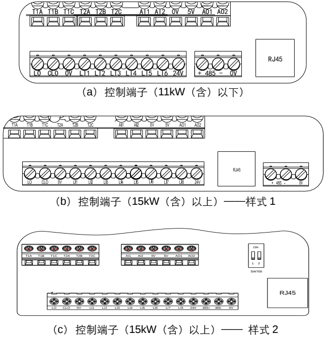
图 4.8 控制端子结构示意图
