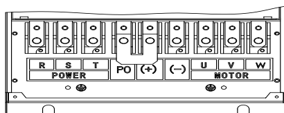
(d) 主回路功率端子 (45kW)
