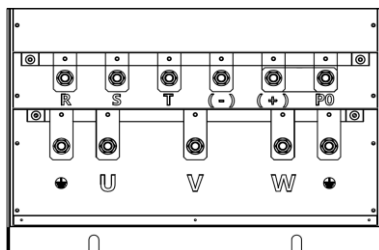
(h) 主回路功率端子 (350-500kW)
