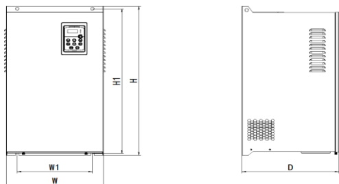
图 3.4 外形及安装尺寸示意图（三相 15KW-45KW）
