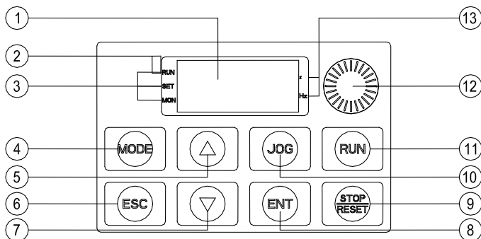
图 5.1 操作面板外形
