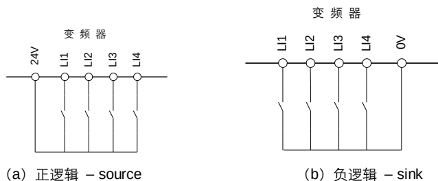
图 4.9 逻辑输入端子接线图
