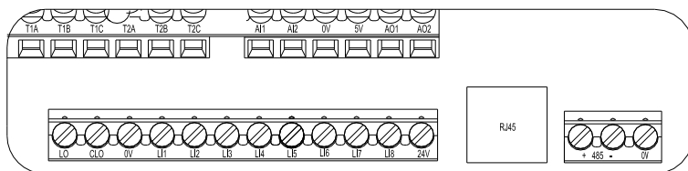
(b) 控制端子 (15kW (含) 以上)
