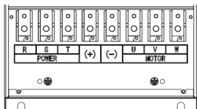
(e) 主回路功率端子 (55kW)
