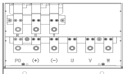
(g) 主回路功率端子 (200-315kW)
