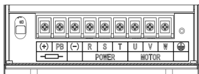
(c) 主回路功率端子 (30-37kW)
