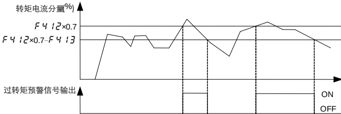
a) 过转矩/过电流报警输出示意图
