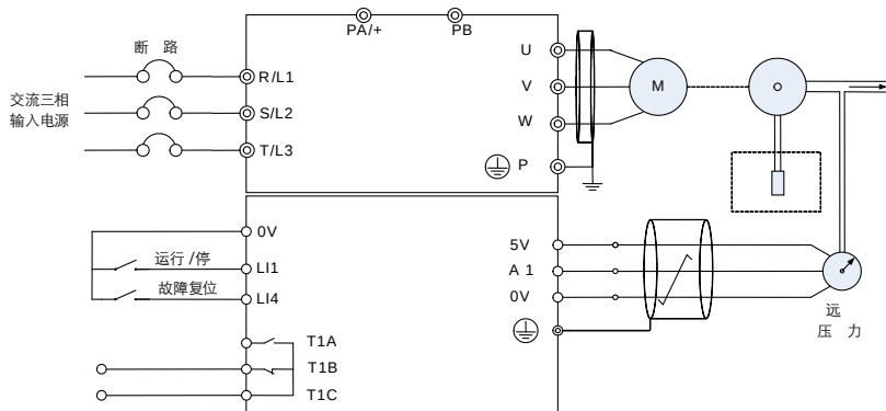
图 5.38 PID 外部连接示例
