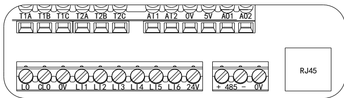
(a) 控制端子 (11kW (含) 以下)
