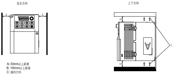
图 4.2 单台安装间距要求
