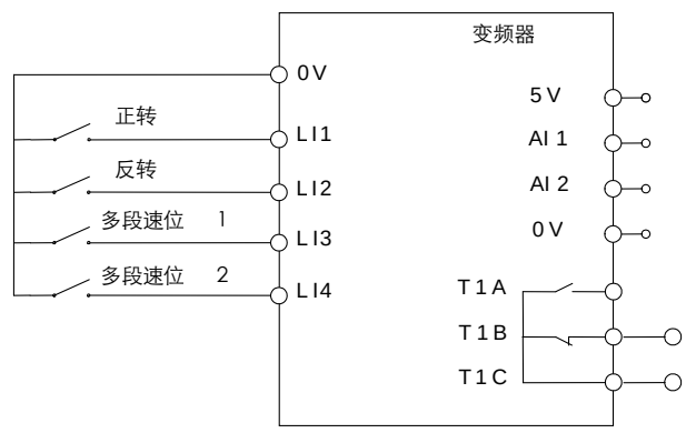
图 5.10 多段速控制接线示意图
