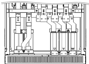
(i) 主回路功率端子 (560-800kW)
