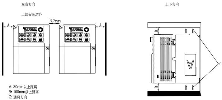
图 4.3 多台左右安装间距要求
