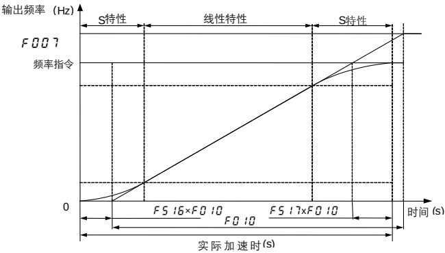
图 6.28 S 型曲线 1
