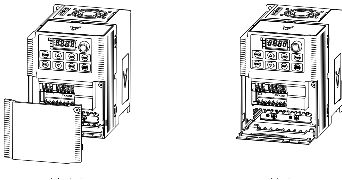
图 4.4 盖板、出线板的拆卸示意图
