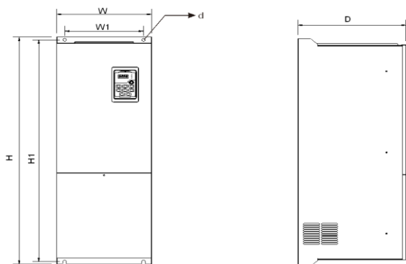
图 3.5 外形及安装尺寸示意图（三相 55KW-500KW）
