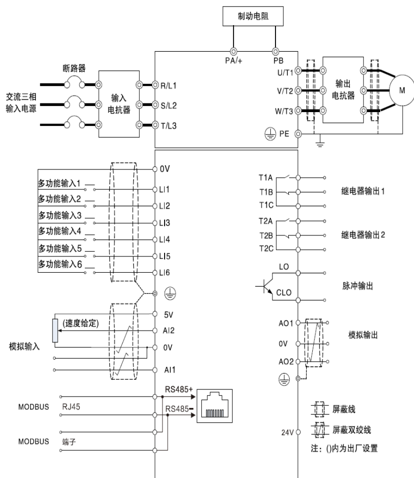
(a) 11kW (含) 以下标准接线图
