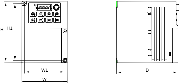
图 3.3 外形及安装尺寸图（三相 11kW（含）以下）
