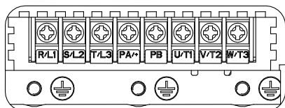
(a) 主回路功率端子 (11kW (含) 以下)
