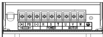
(b) 主回路功率端子 (15-22kW)
