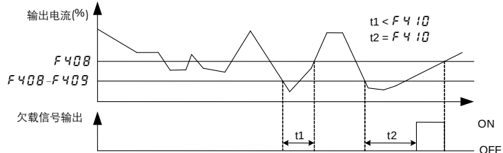
图 6.21 欠载信号输出示意图
