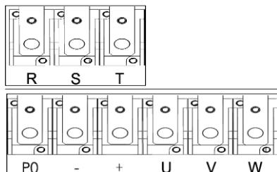
(f) 主回路功率端子 (75-185kW)
