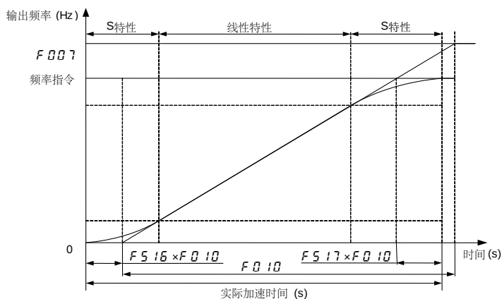
图 5.28 S 型曲线 1
