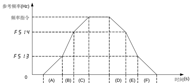
图 5.30 加减速曲线的自动切换
