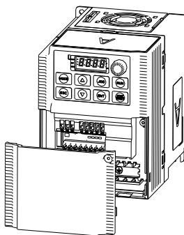
(A)拆卸盖板
