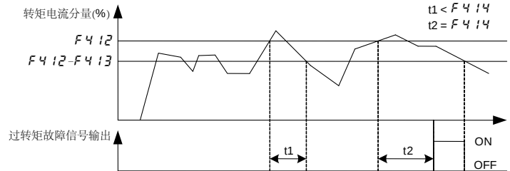
b) 过转矩故障输出信号示意图
