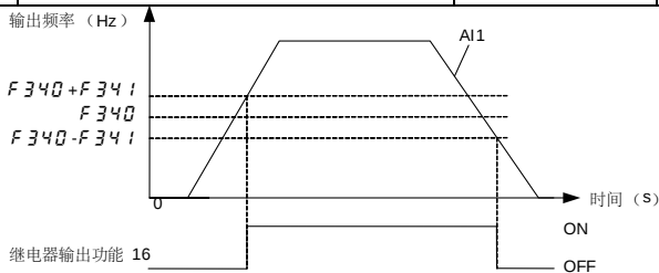
图 5.15 继电器输出-AI1 输入检出示意图
