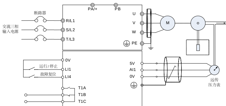
图 5.38 PID 外部连接示例
