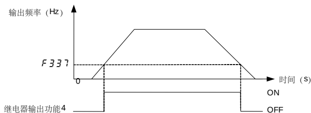
图 5.13 继电器输出-低速频率检出示意图
