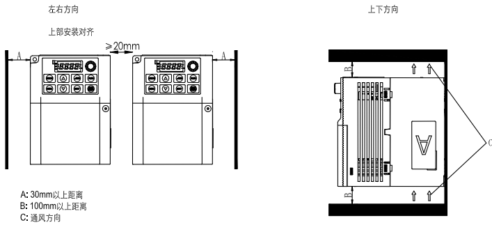
图 3.3 多台左右安装间距要求
