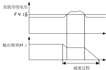
图 5.23 过压故障工作电平示意
