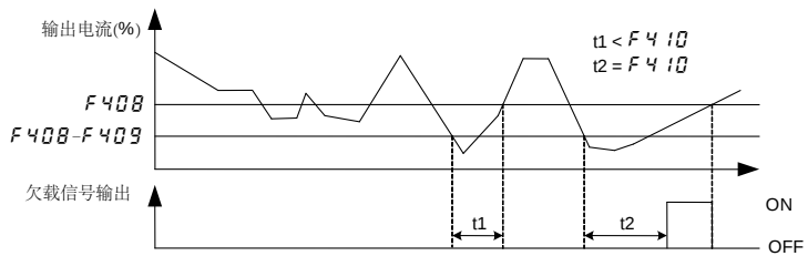
图 5.21 欠载信号输出示意图
