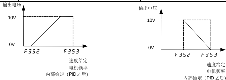
图 5.19 F352 和 F353 设路示意图
