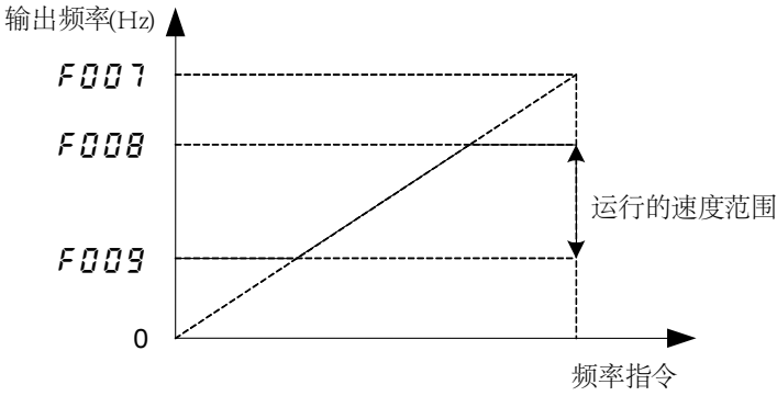
图 5.2 F007 , F008 , F009 和运行速度关系
