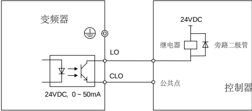
图 5.9 集电极逻辑输出接线示意图
