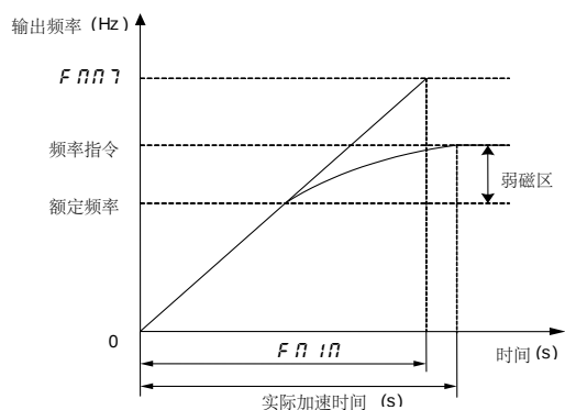
图 5.29 S 型曲线 2
