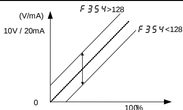
图 5.20 模拟输出曲线与 F354 关系
