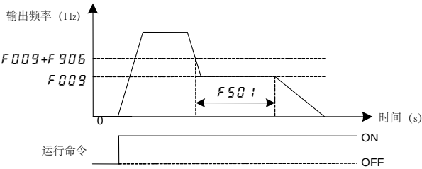
图 5.25 休眠模式进入
