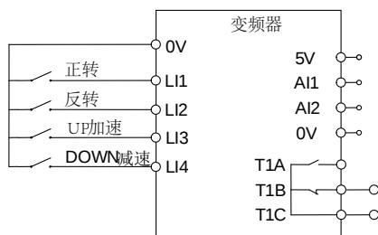
图 4.10 UP/DOWN 加减速接线示意图
