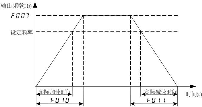
图 5.3 加速时间和减速时间定义
