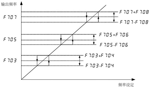
图 5.34 跳跃频率参数设略示意
