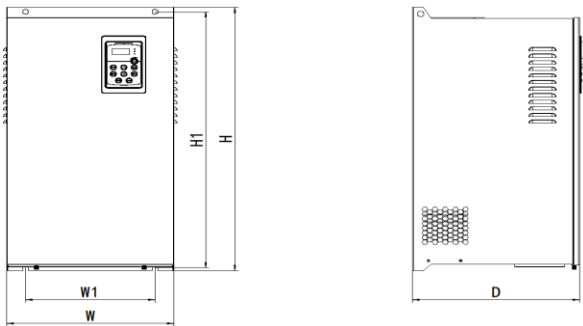
图 2.5 外形及安装尺寸示意图（三相 18.5kW（含）以上）
