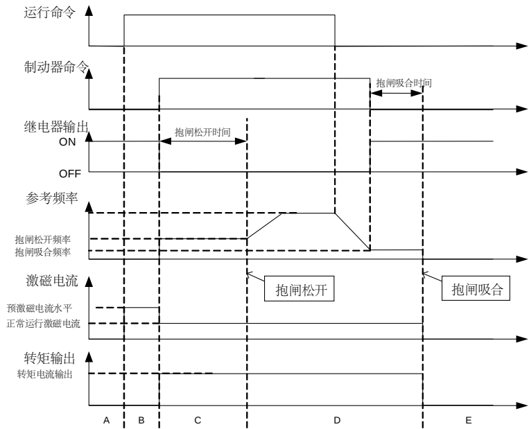
图 5.35 制动器逻辑时序示意图
