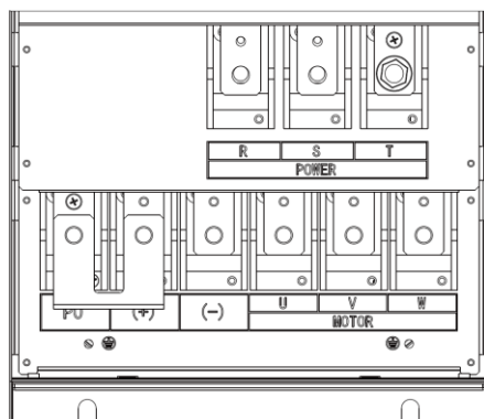
(f) 主回路功率端子 (160-185kW)
