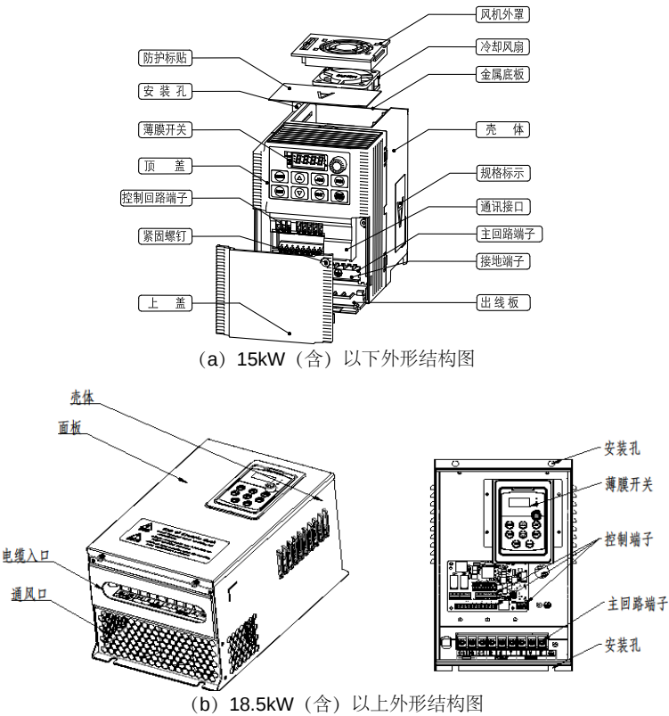
图 2.3 外形结构图
