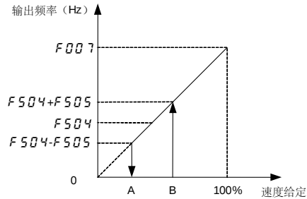
图 5.26 运行起始频率
