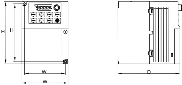
图 2.4 外形及安装尺寸图（单相、三相 15kW（含）以下）
