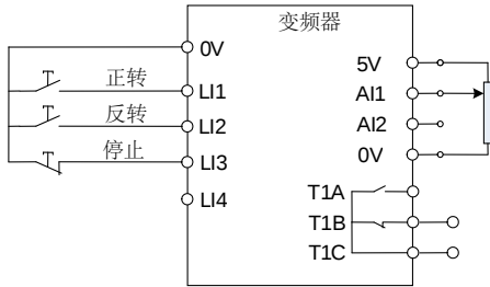
图 4.8 3 线控制（负逻辑、减速停机）接线示意图
