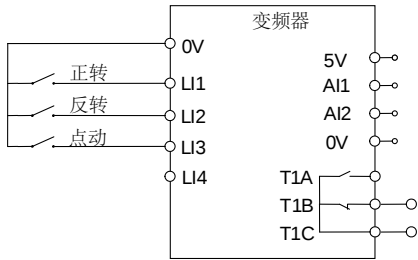
图 4.12 点动控制接线示意图
