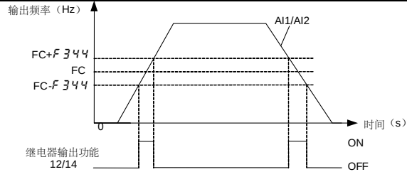
图 5.17 继电器输出-速度给定等于 AI1 / AI2 信号
