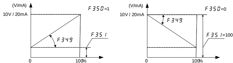
图 5.18 参数 F349 , F350 和 F351 设路示意图
