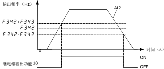
图 5.16 继电器输出-AI2 输入检出示意图
