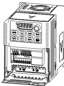
(B)拆卸出线板
