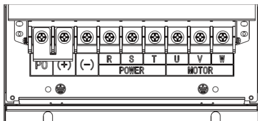
(d) 主回路功率端子 (55-75kW)
