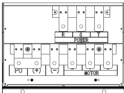
(g) 主回路功率端子 (200-250kW) 壁挂式
