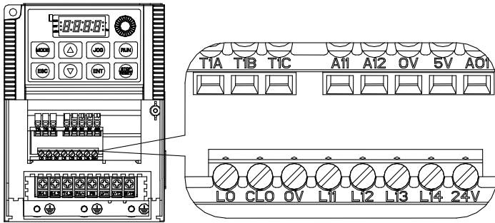
(b) 控制端子（15kW（含）以下）
