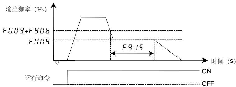
图 5.40 休眠模式进入
