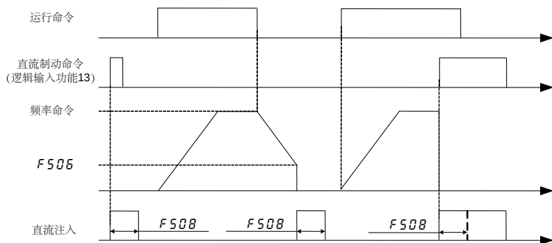
图 5.27 直流制动时序
