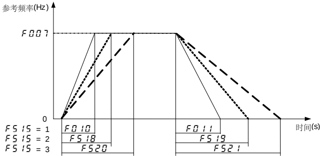
图 5.31 加/减速时间参数
