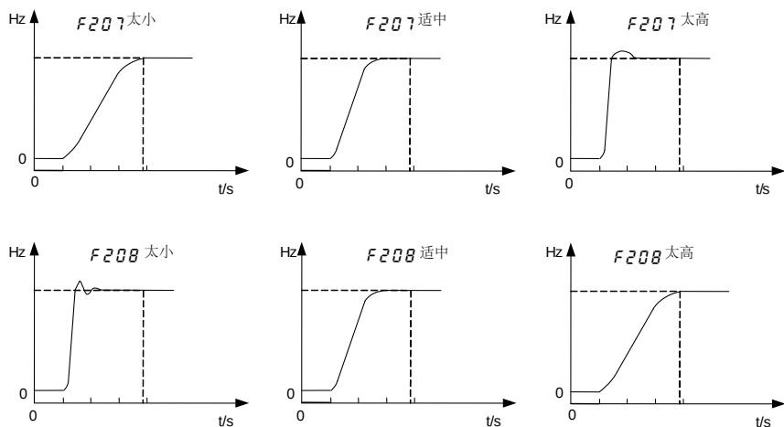
图 5.6 速度环参数与速度响应关系
