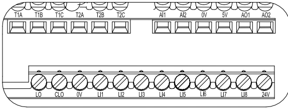
(a) 控制端子（18.5kW（含）以上）
