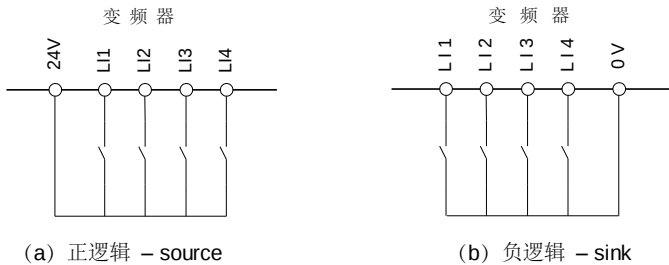
图 3.9 逻辑输入端子接线图
