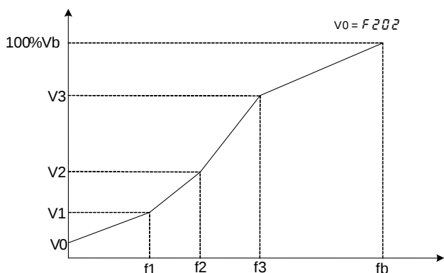
图 5.7 多点 V/f 控制( F217=2 )
