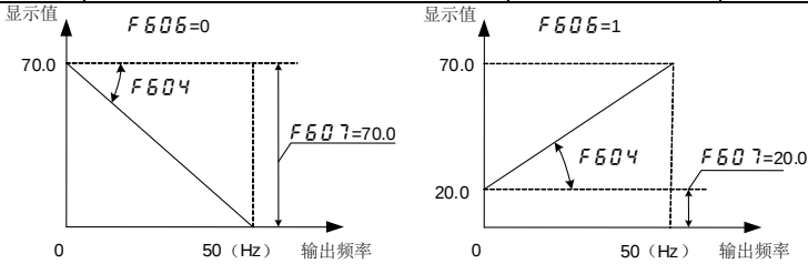
图 5.33 定制频率显示示意图
