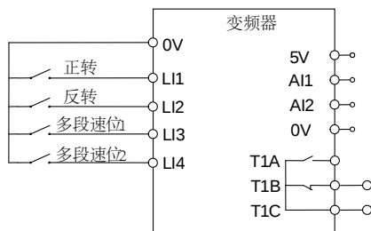
图 4.11 多段速控制接线示意图
