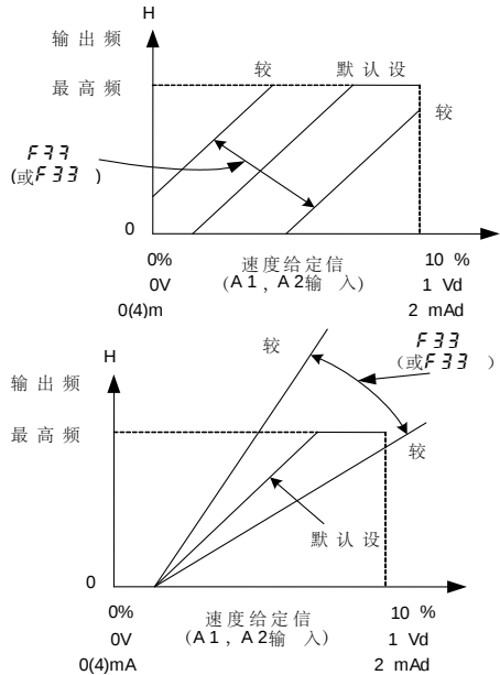
图 5.12 模拟输入校准
