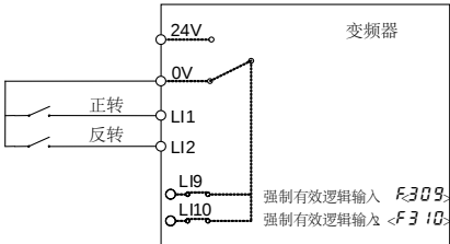
图 5.8 强制有效逻辑输入功能
