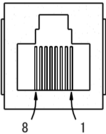
图 A.1 RJ45 正视图
