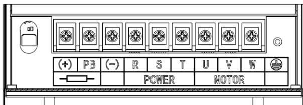
(c) 主回路功率端子 (37-45kW)
