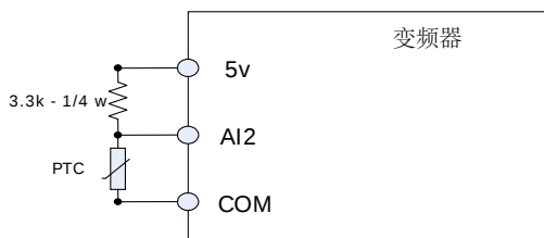
图 5.24 PTC 接线示例
