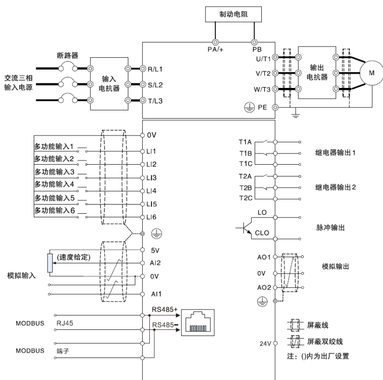
(b) 15kW (含) 以下标准接线图
