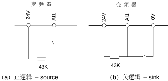
图 3.8 AI1 配路为逻辑输入端子时的接线图
