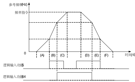
图 5.32 通过逻辑输入切换加速/减速曲线
