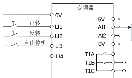
(3) 远程模式示例 3: 3 线控制（负逻辑，自由停机）
