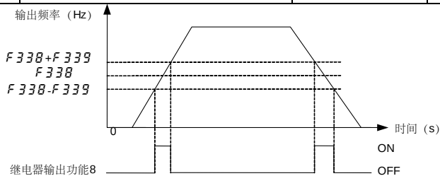
图 5.14 继电器输出-频率检出 2 示意图
