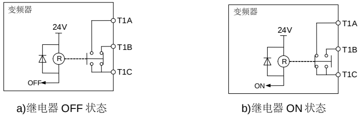
图 5.10 继电器状态说明
