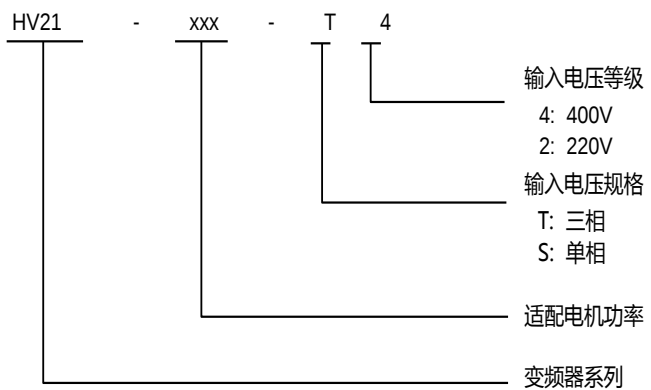
图 2.2 变频器型号说明示意图
