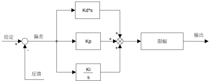
图 5.37 PID 调节器框图
