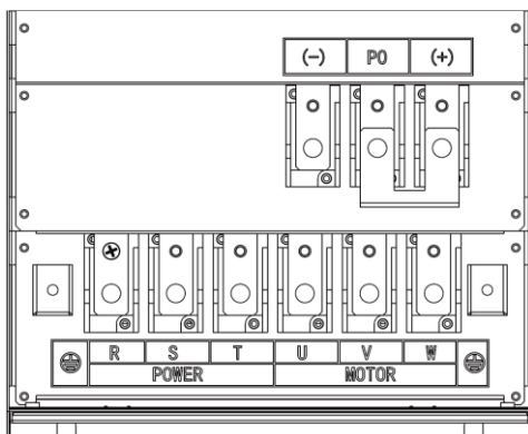
(e) 主回路功率端子 (90-132kW)
