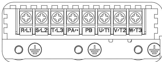
(a) 主回路功率端子 (15kW (含) 以下)
