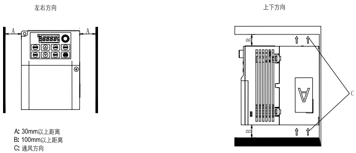
图 3.2 单台安装间距要求
