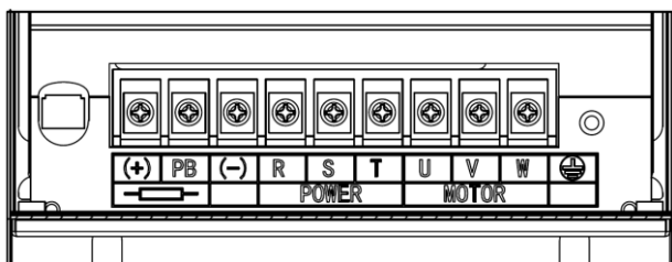
(b) 主回路功率端子 (18.5-30kW)
