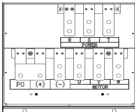
(h) 主回路功率端子 (280-355kW)
