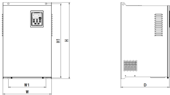
图 3.4 外形及安装尺寸示意图（三相 15KW-315KW）
