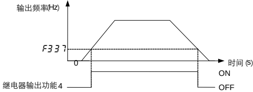
图 6.13 继电器输出-频率检出示意图
