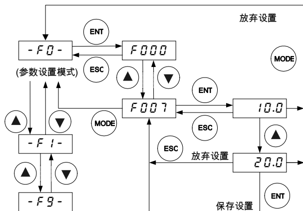
图 5.4 参数设置模式导航
