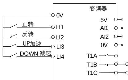
图 5.9 UP/DOWN 加减速接线示意图
