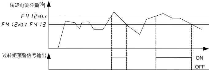
a) 过转矩/过电流报警输出示意图
