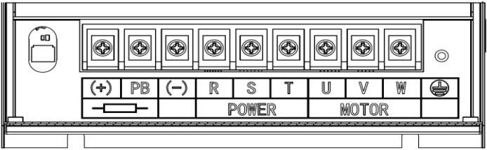
(d) 主回路功率端子（30-37kW）
