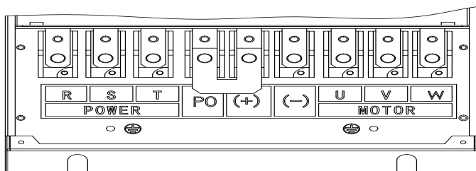
(e) 主回路功率端子 (45kW)
