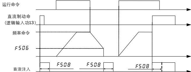
图 6.27 直流制动时序
