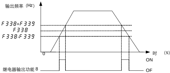
图 6.14 继电器输出-频率检出 2 示意图
