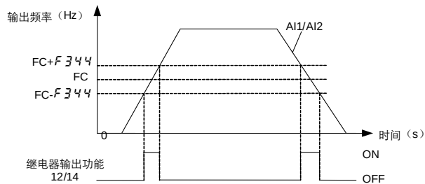
图 6.17 继电器输出-AI1/AI2 输入检出示意图
