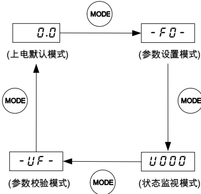
图 5.2 变频器模式切换示意图
