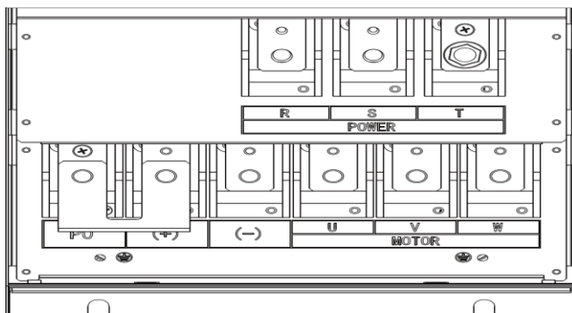
(h) 主回路功率端子 (132-185kW)
