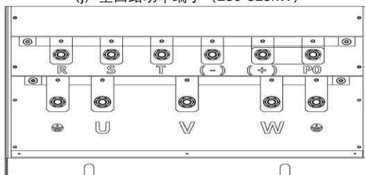
(k) 主回路功率端子 (355-500kW)
