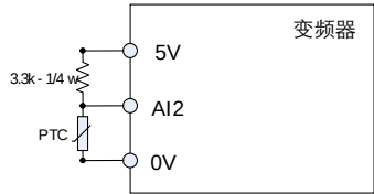
图 6.24 PTC 接线示例
