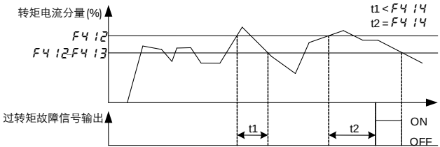
b) 过转矩/过电流故障输出信号示意图
