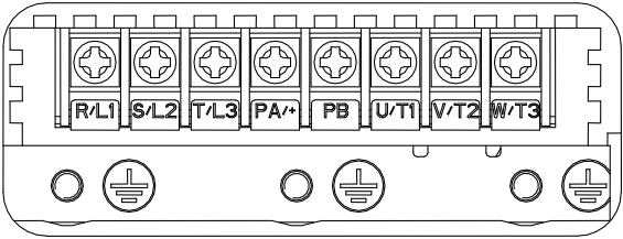
(a) 主回路功率端子（11kW（含）以下）
