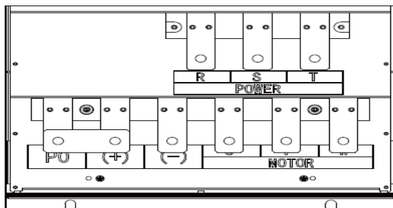
(i) 主回路功率端子 (200-220kW)
