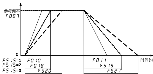
图 6.31 加/减速时间参数
