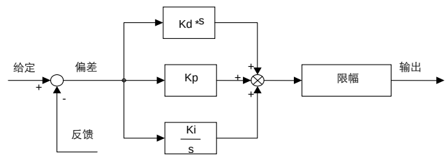
图 6.37 PID 调节器框图
