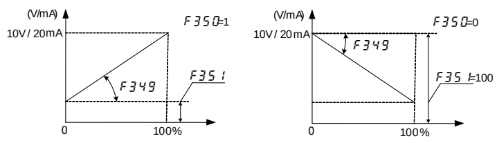
图 6.18 参数 F349 , F350 和 F351 设置示意图
