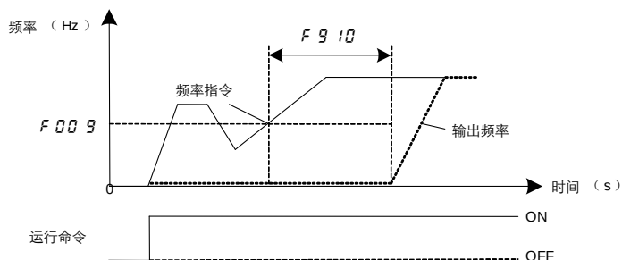
图 6.39 休眠唤醒示意图
