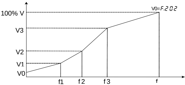
图 6.7 多点 V/f 控制( F2 17 =2)
