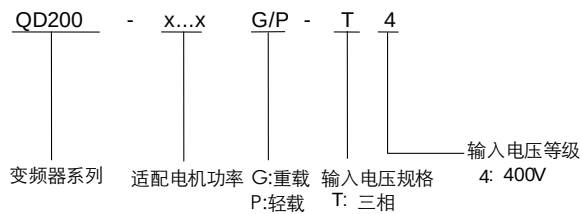
图 3.1 变频器型号说明示意图
