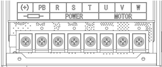
(b) 主回路功率端子（15-18.5kW）
