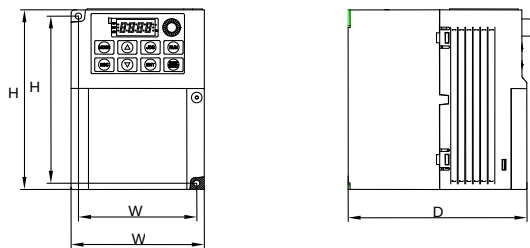
图 3.3 外形及安装尺寸图（三相 11kW（含）以下）
