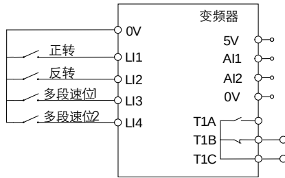
图 5.10 多段速控制接线示意图
