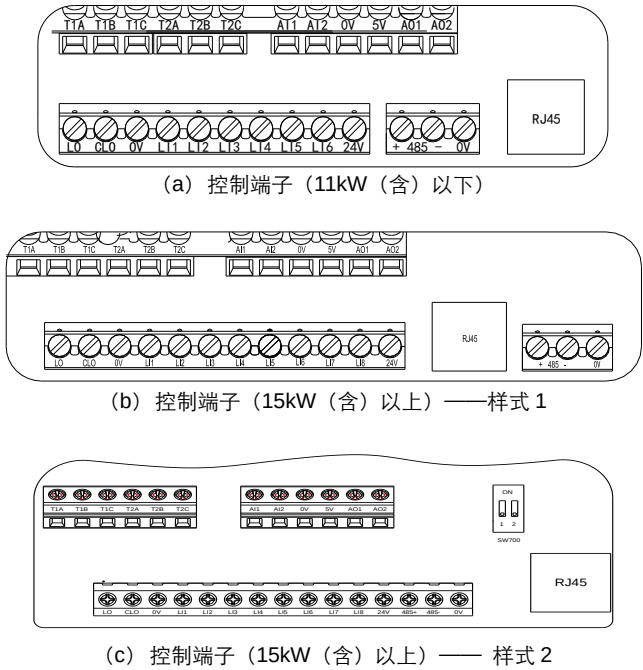
图 4.7 控制端子结构示意图
