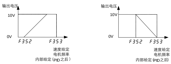
图 6.19 F352 和 F353 设置示意图
