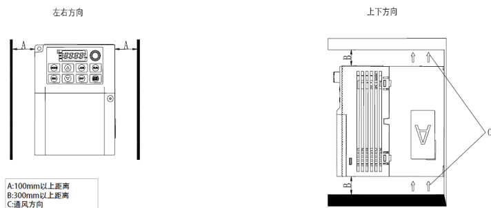
图 4.2 单台安装间距要求
