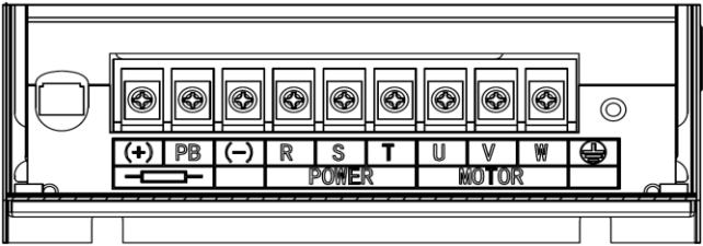
(c) 主回路功率端子（22kW）
