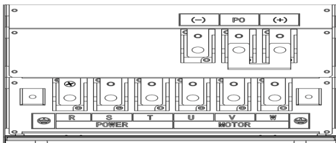
(g) 主回路功率端子 (75-110kW)
