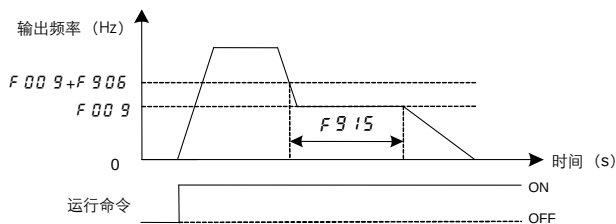
图 6.40 休眠模式进入
