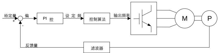
图 6.36 PID 控制基本原理框图
