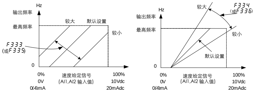
图 6.12 模拟输入校准
