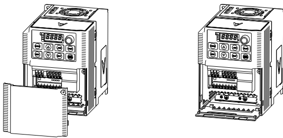
图 4.4 盖板、出线板的拆卸示意图
