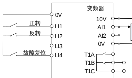
图 5.7 2 线控制接线示意图
