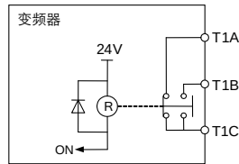
b)继电器 ON 状态
