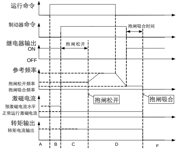
图 6.35 制动器逻辑时序示意图
