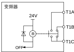
a)继电器 OFF 状态
