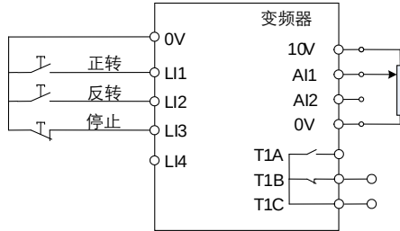
图 5.8 3 线控制（负逻辑）接线示意图
