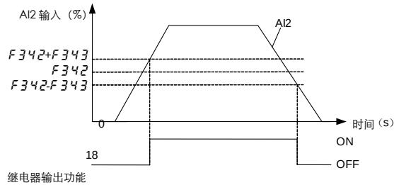
图 6.16 继电器输出-AI2 输入检出示意图
