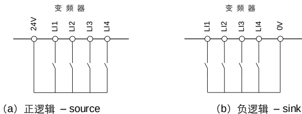
图 4.9 逻辑输入端子接线图
