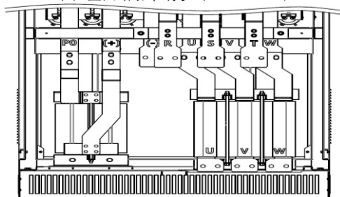
(l) 主回路功率端子 (560-800kW)
