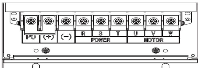
(f) 主回路功率端子 (55kW)
