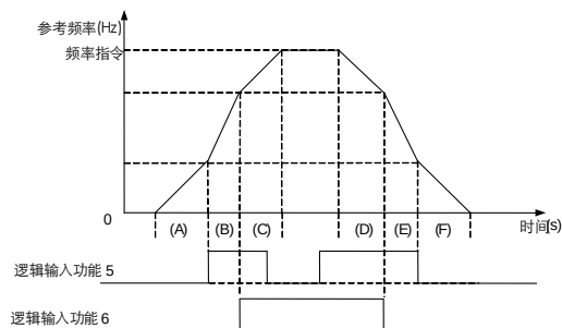
图 6.32 通过逻辑输入切换加减速曲线
