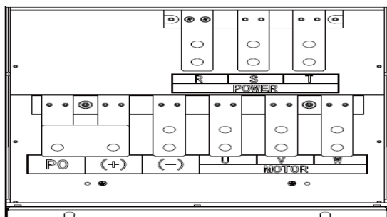
(j) 主回路功率端子 (250-315kW)
