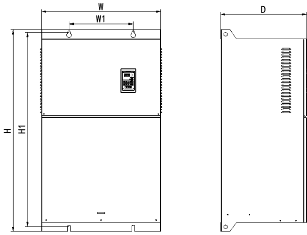
图 3.5 外形及安装尺寸示意图（三相 355KW-500KW）
