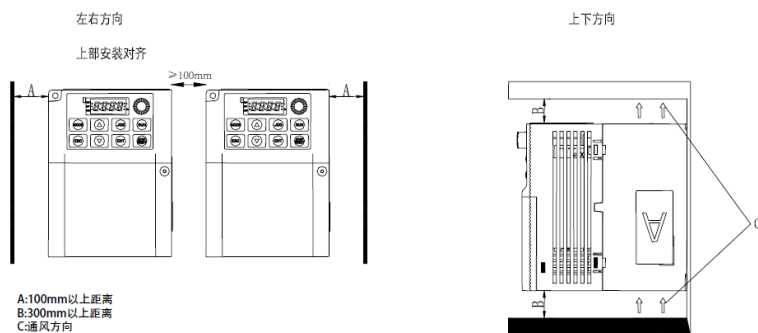
图 4.3 多台左右安装间距要求
