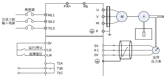
图 6.38 PID 外部连接示例
