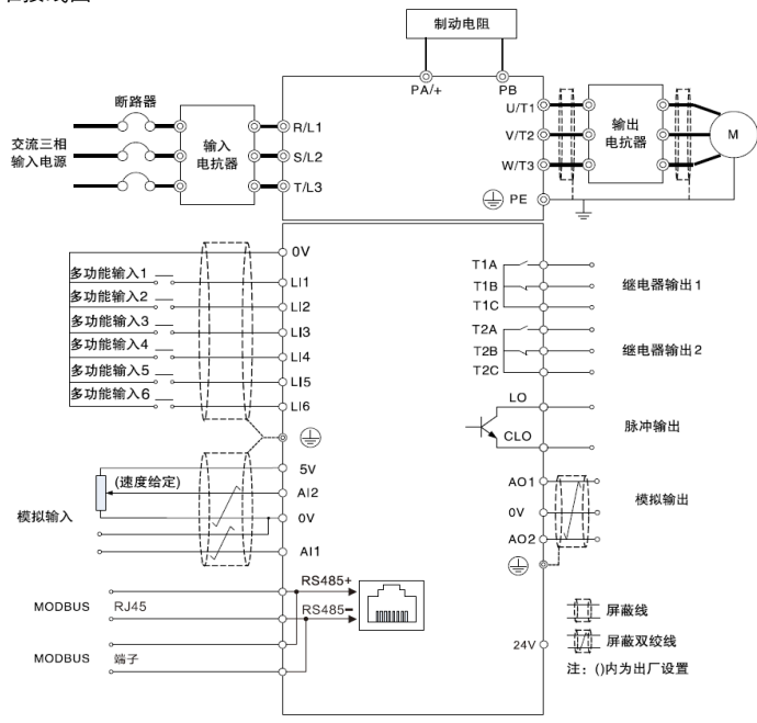
(a) 11kW（含）以下标准接线图
