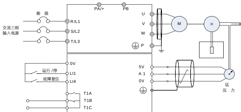
图 6.41 PID 外部连接示例
