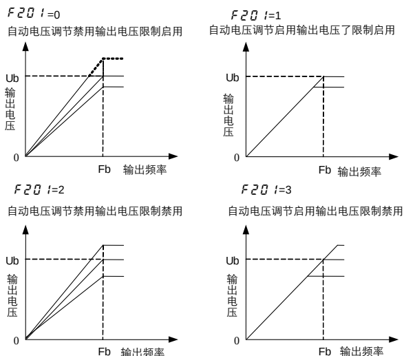
图 6.5 AVR 功能示意图
