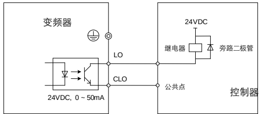
图 6.9 集电极逻辑输出接线示意图
