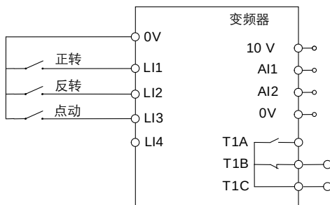
图 5.11 点动控制接线示意图
