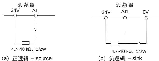
图 4.8 AI1 配置为逻辑输入端子时的接线图
