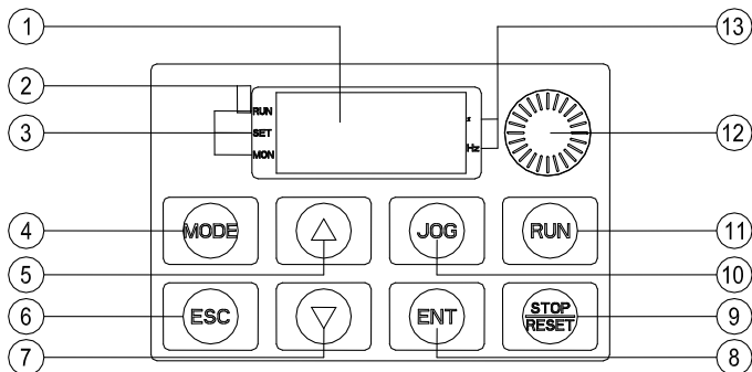
图 5.1 操作面板外形
